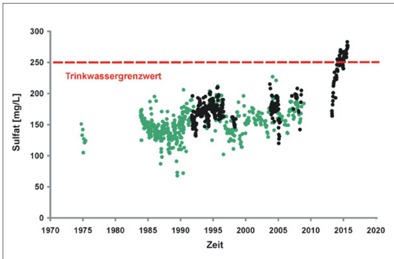
Sulfatkonzentrationen im Müggelsee von 1975-2015 (schwarz: unveröffentlichte Langzeitdaten des IGB; grün: Daten der Senatsverwaltung für Stadtentwicklung und Umwelt Berlin)
